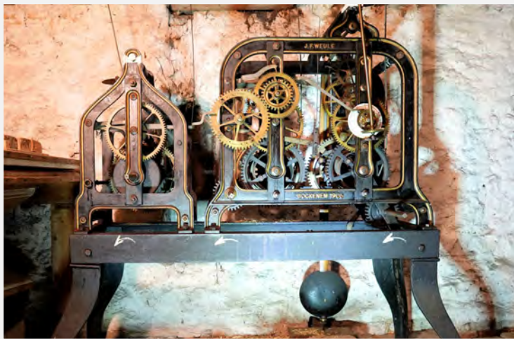
Das Uhrwerk der Turmuhr der Firma Weule von 1905
